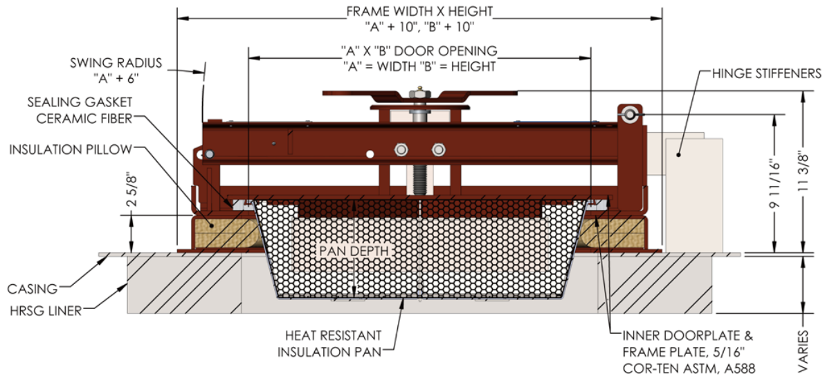
DOOR TYPE BM FOR HRSG
